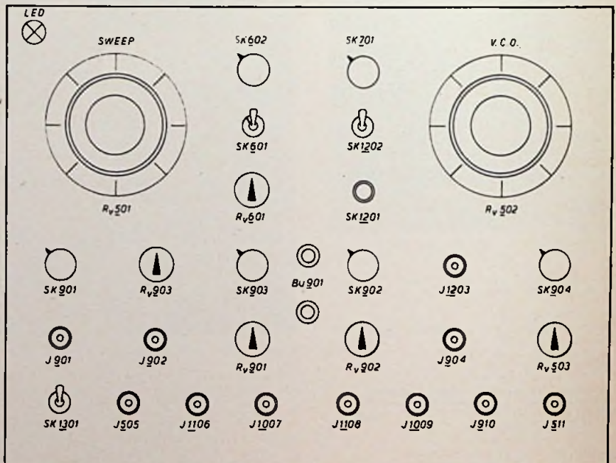
Fig. 15. Positie van de bedieningsorganen. Het eerste cijfer geeft het fig. nummer aan waar het betreffende onderdeel is getekend.
